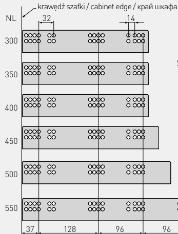
Rozstaw otworów montażowych Mounting dimensions Монтажные отверстия
